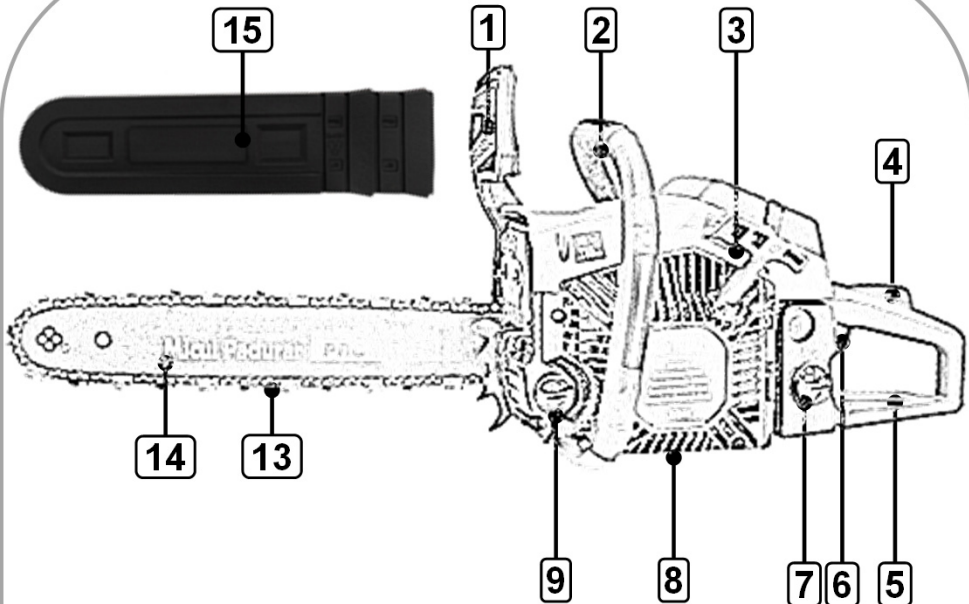
Lista componentelor
